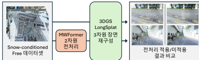
그림 2 : 3DGS의 강설 강건성 연구를 위한 실험 파이프라인
