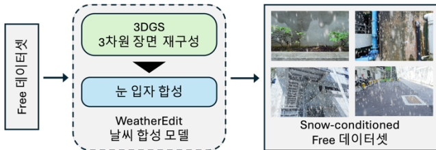
그림 1 : Snow-conditioned Free 데이터셋 구축 파이프라인
